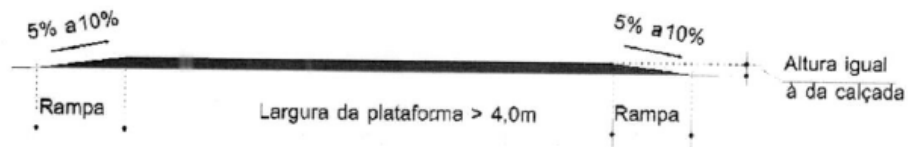
CORTE A-A
