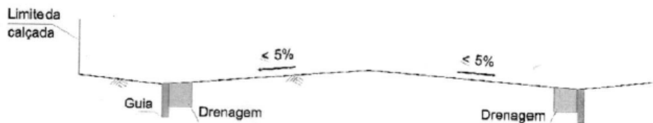
CORTE B-B
